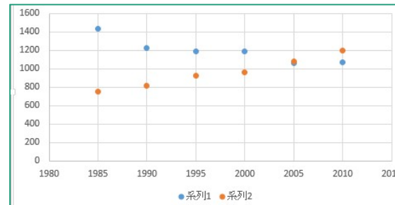
散布図
