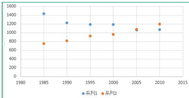
散布図
