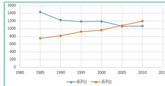
折れ線
