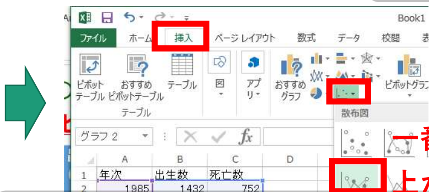
元データ
