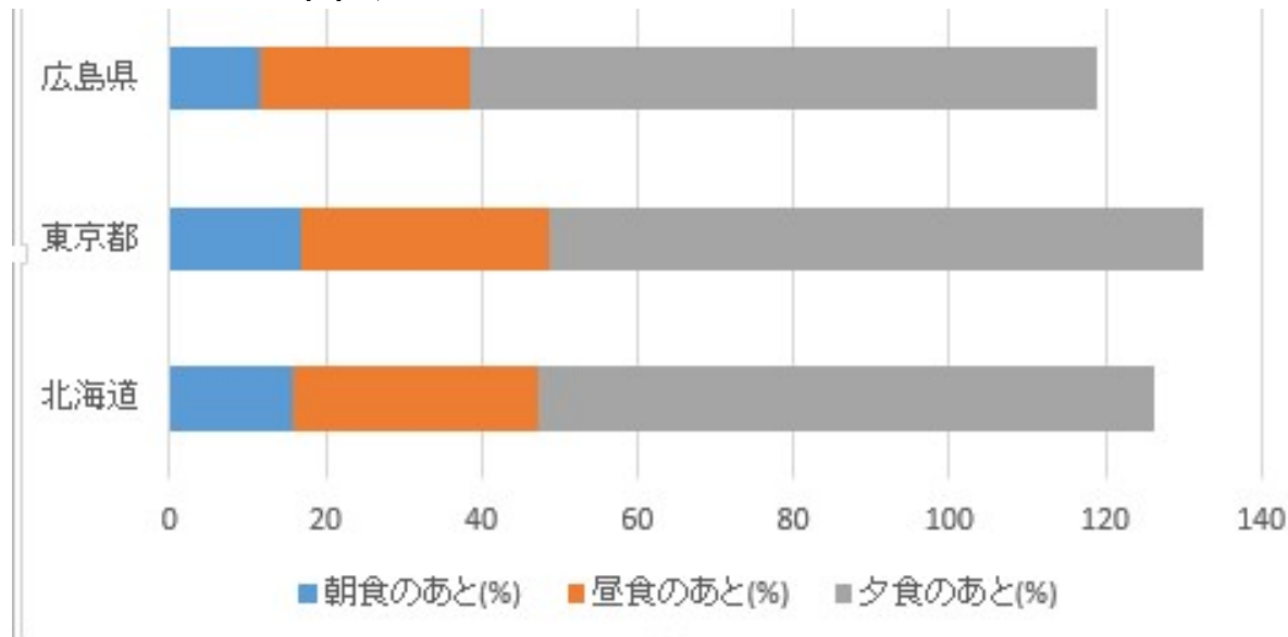
横棒グラフ
