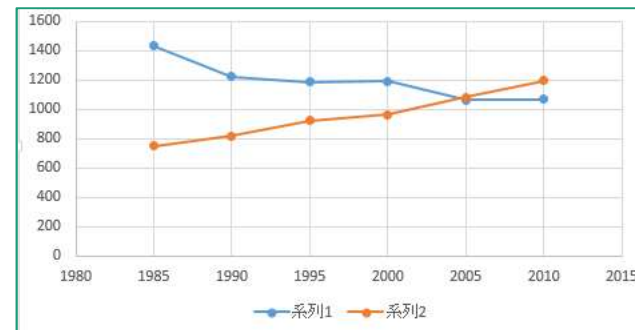
折れ線
