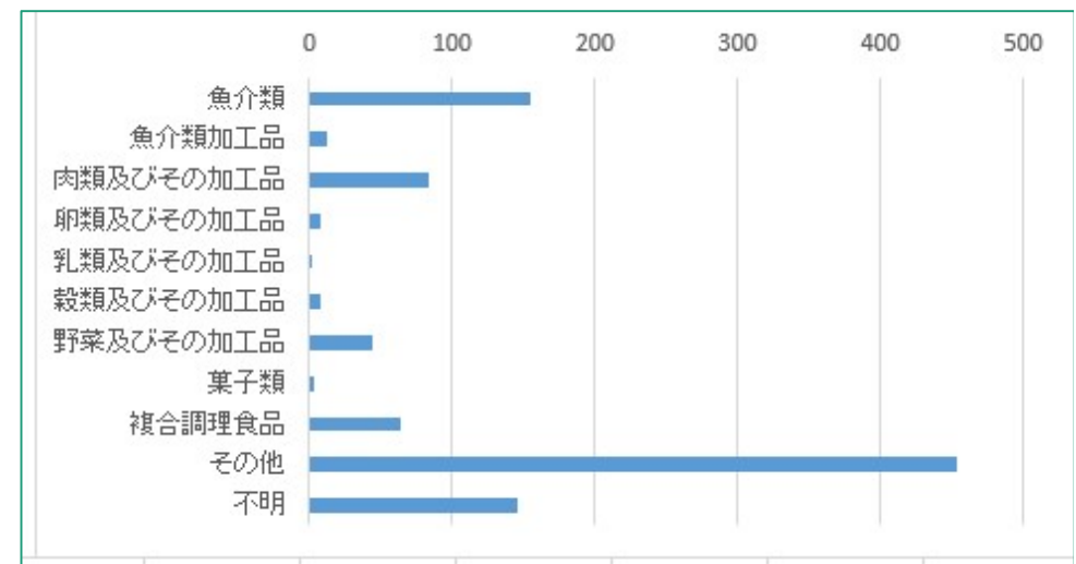
横棒グラフ
